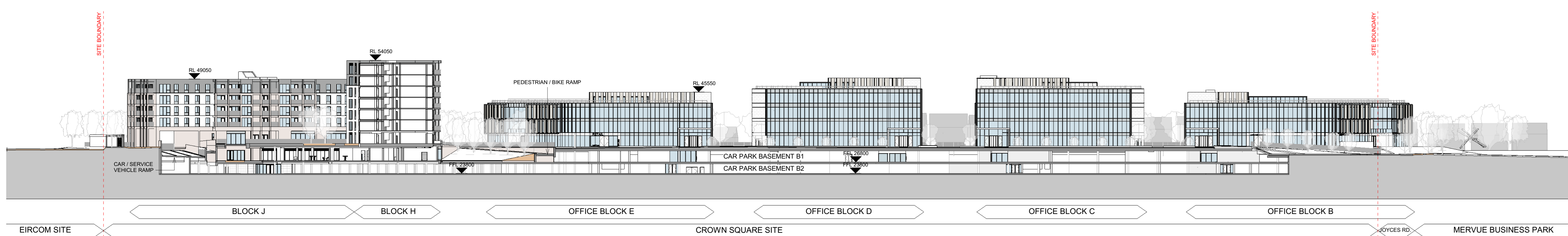
1 Site Section 01 1 : 500
