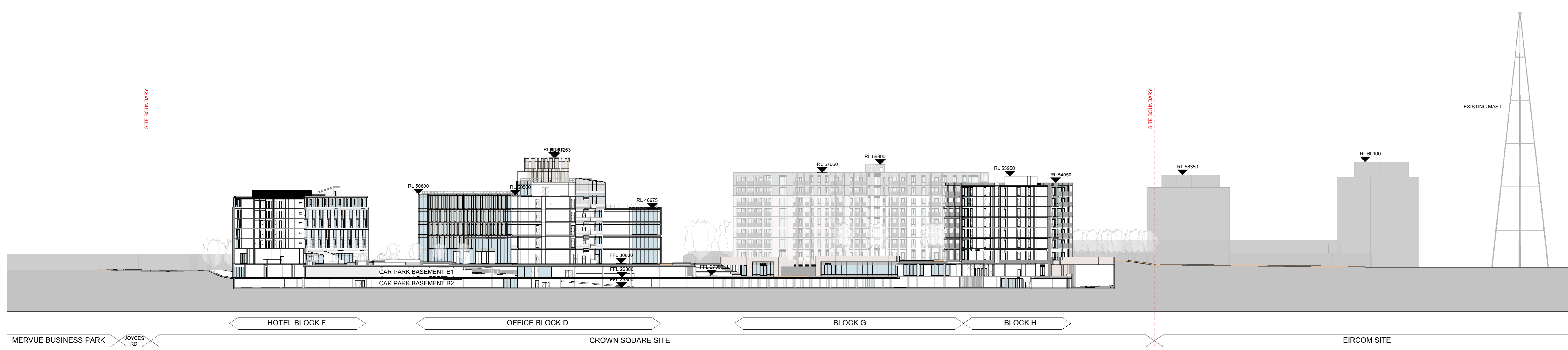
5 Site Section 05 1 : 500
