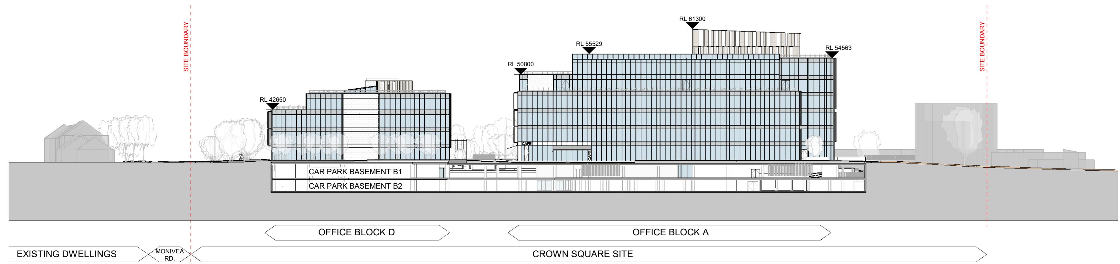
3 Site Section 03 1 : 500
