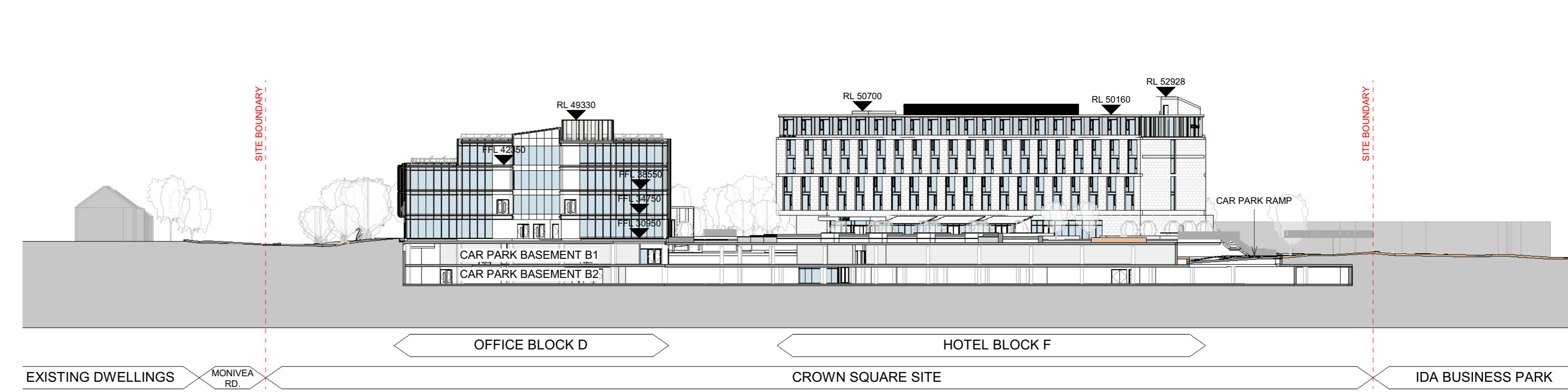
4 Site Section 04 1 : 500
