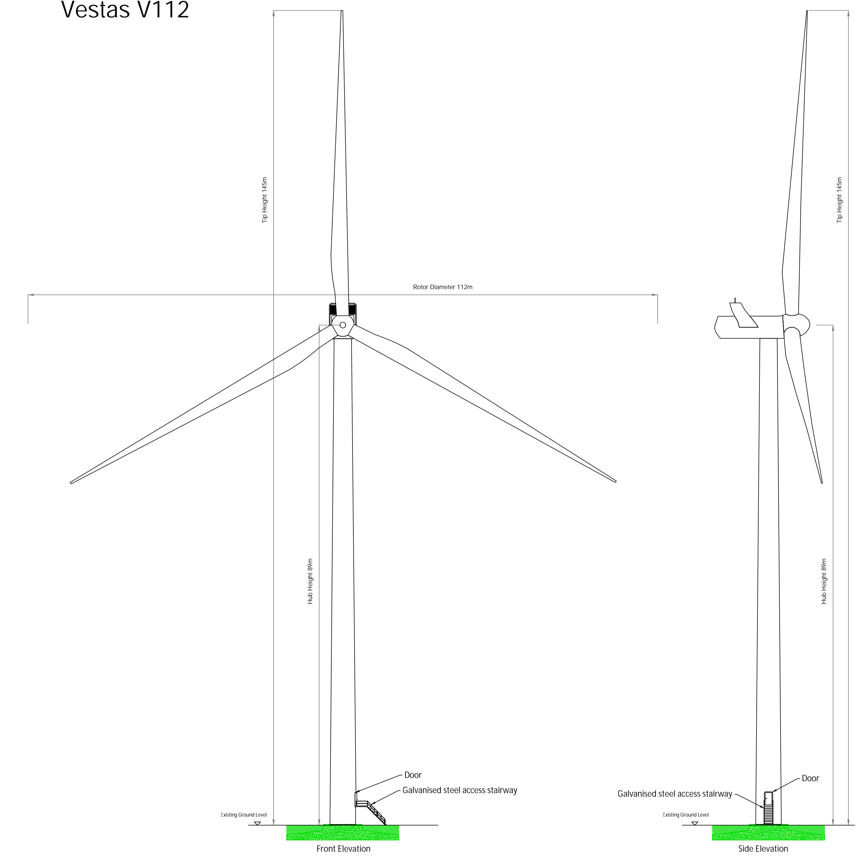
Vestas V112
