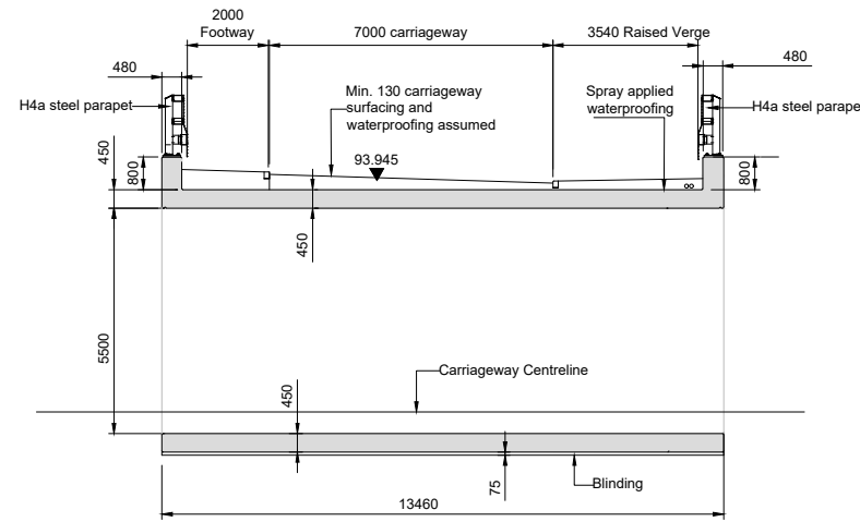
SECTION A Scale 1 : 100
