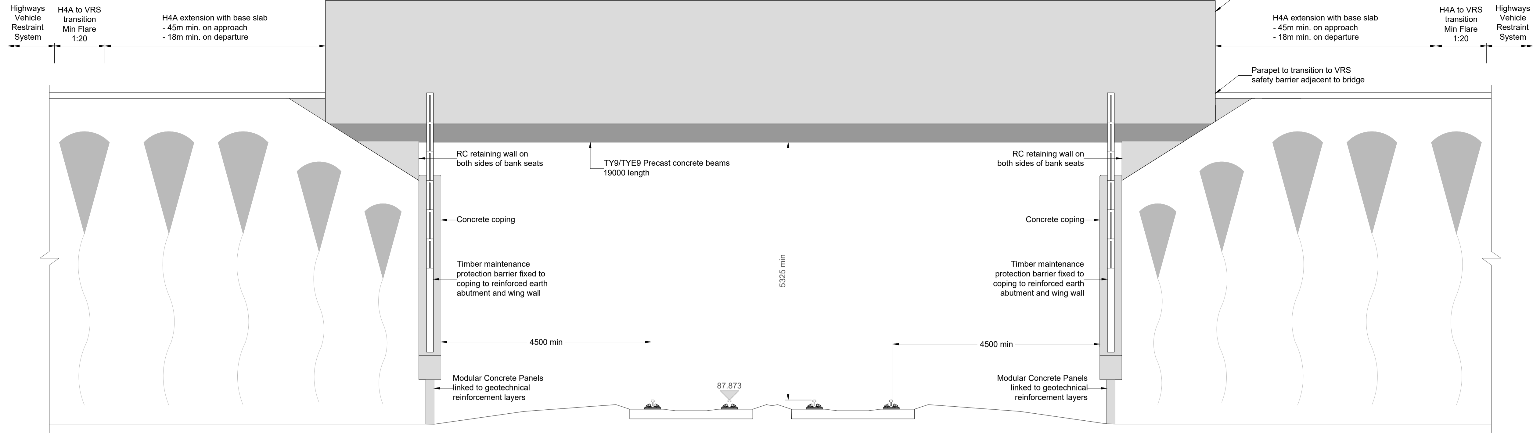
SECTION A Scale 1 : 50 001
