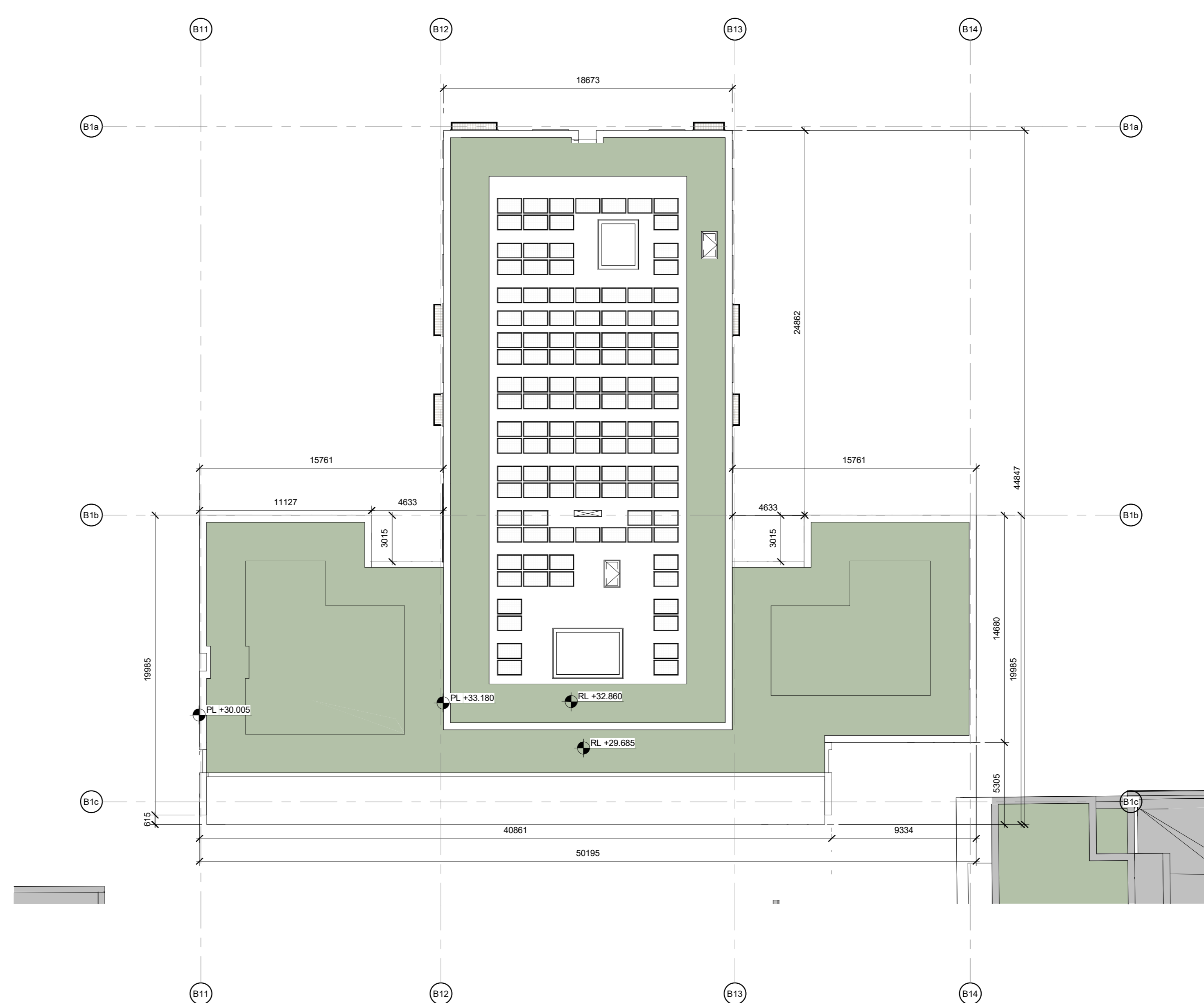
4 ROOF_Z2_FFL 1 : 200
