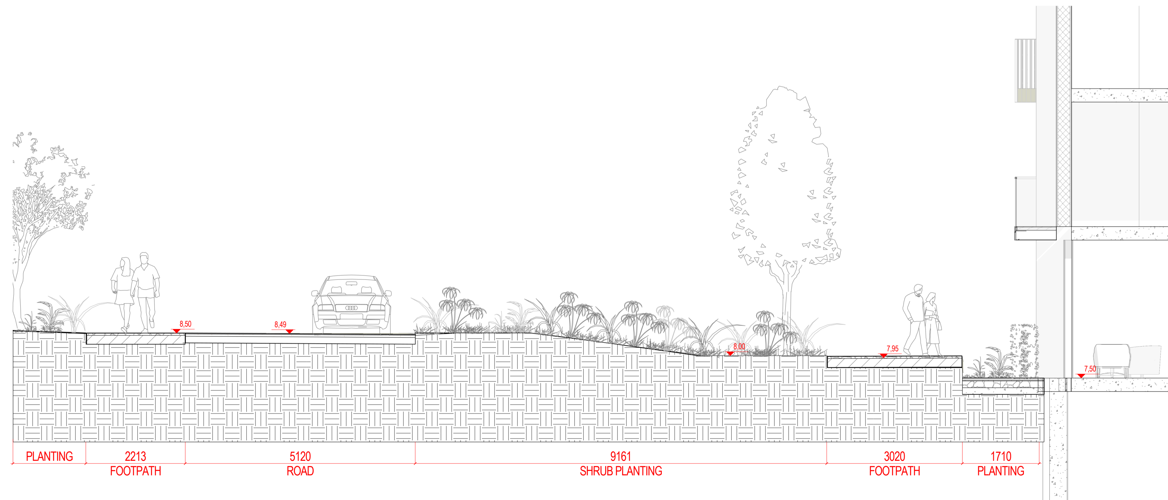
2 SECTION 62 1:50 @A1
