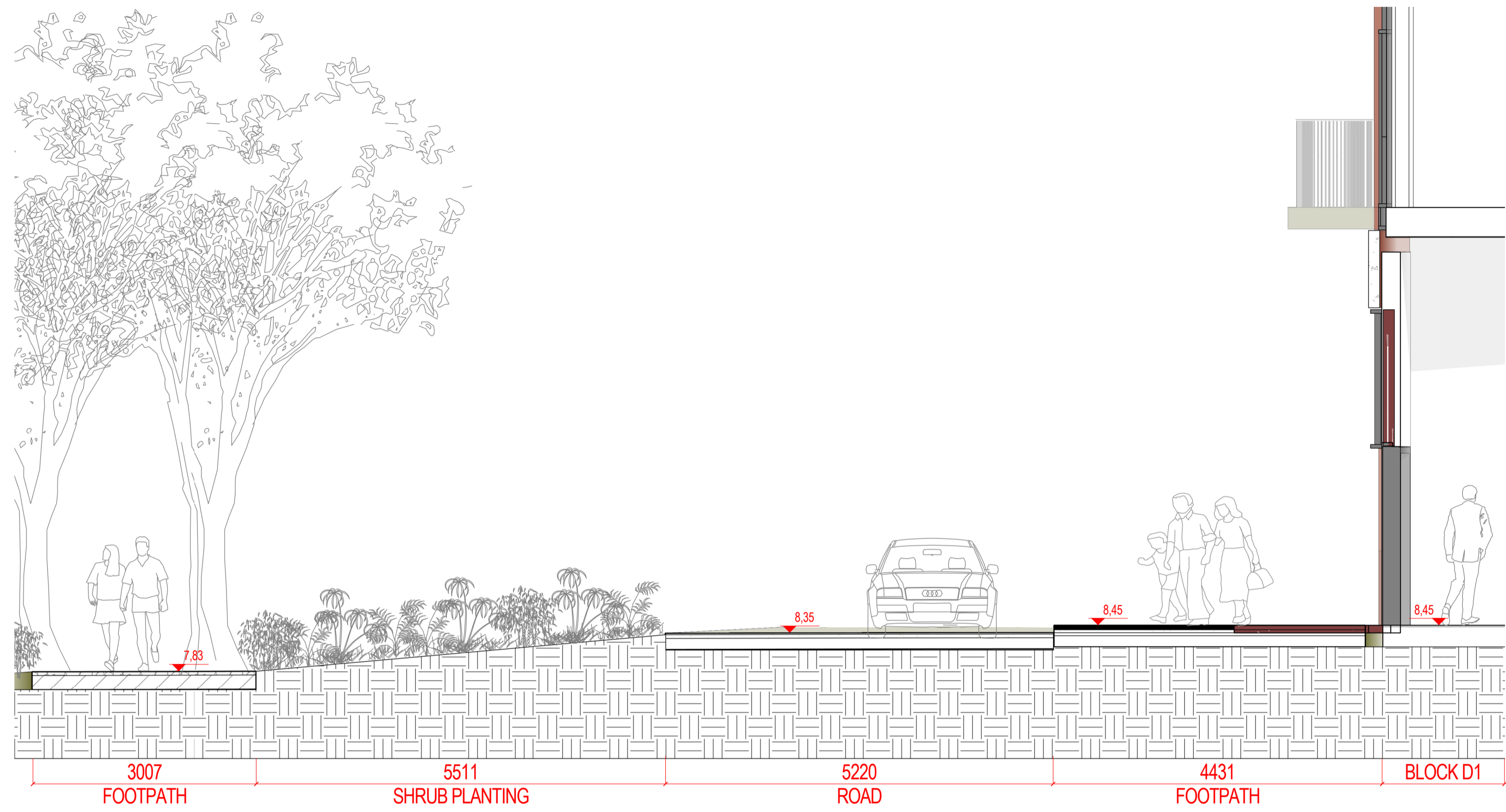
1 SECTION 61 1:50 @A1
