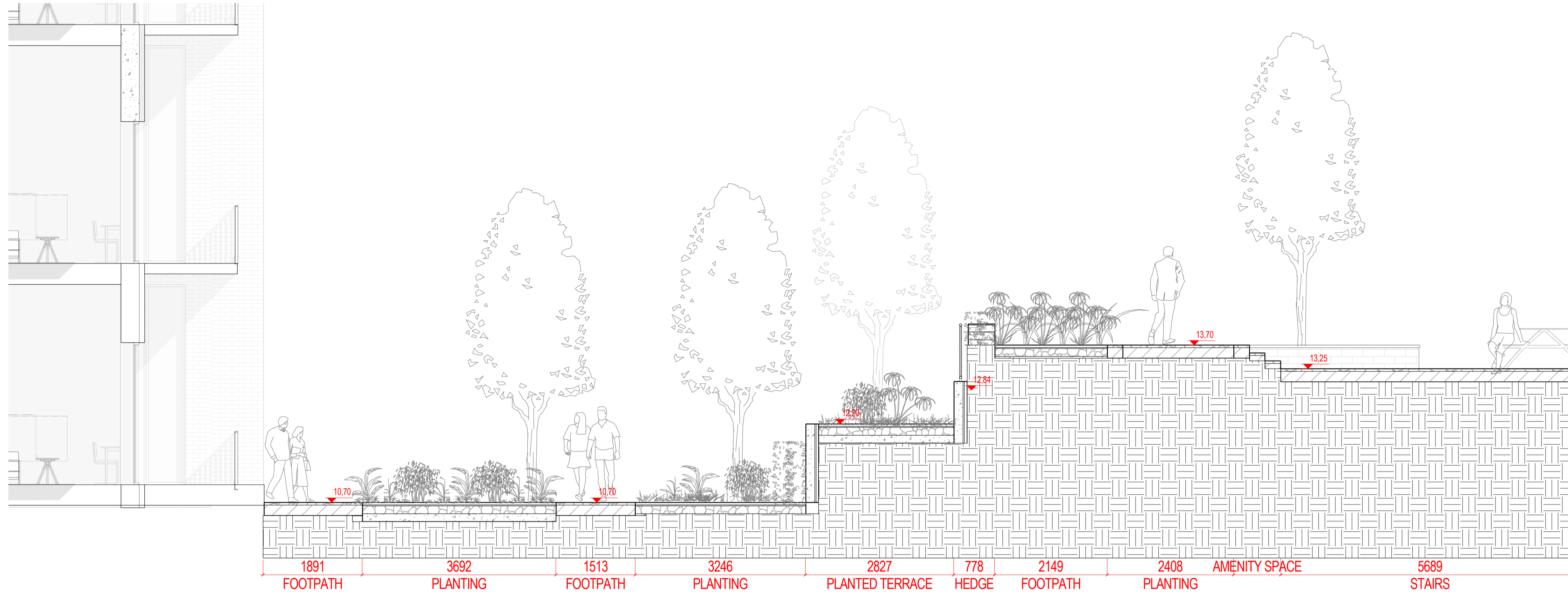
1 SECTION 68 1:50 @A1
