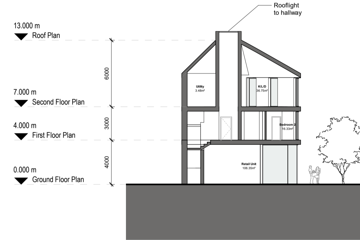
2 Section B_B 1 : 200
