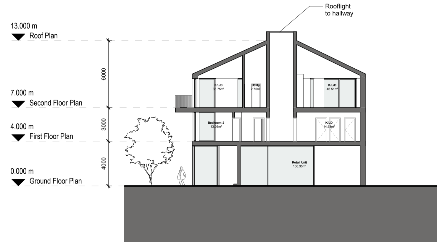
1 Section A_A 1 : 200
