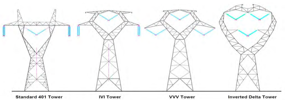
Fíor 3.1: Léaráidí Imlíneacha de na Túir Chruach Laitíse (níl siad de réir scála)
