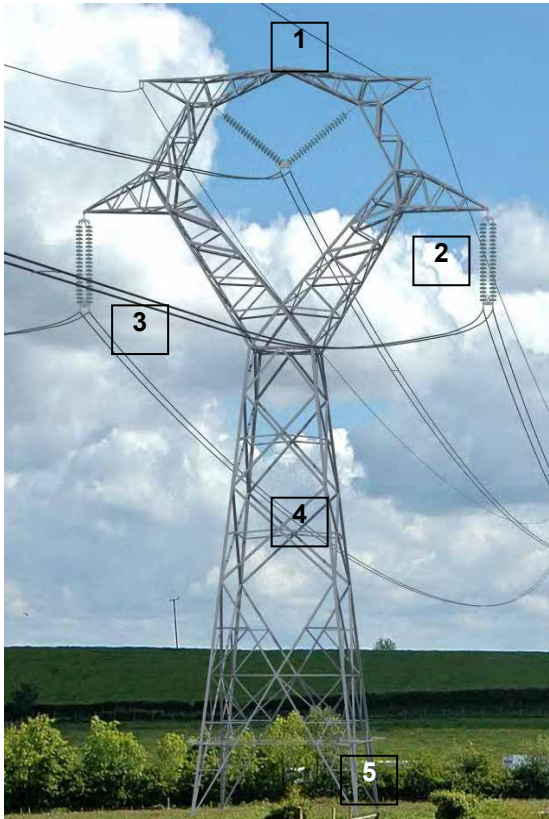
Fíor 4.4: Leagan Amach Ginearálta an Túir IVI
