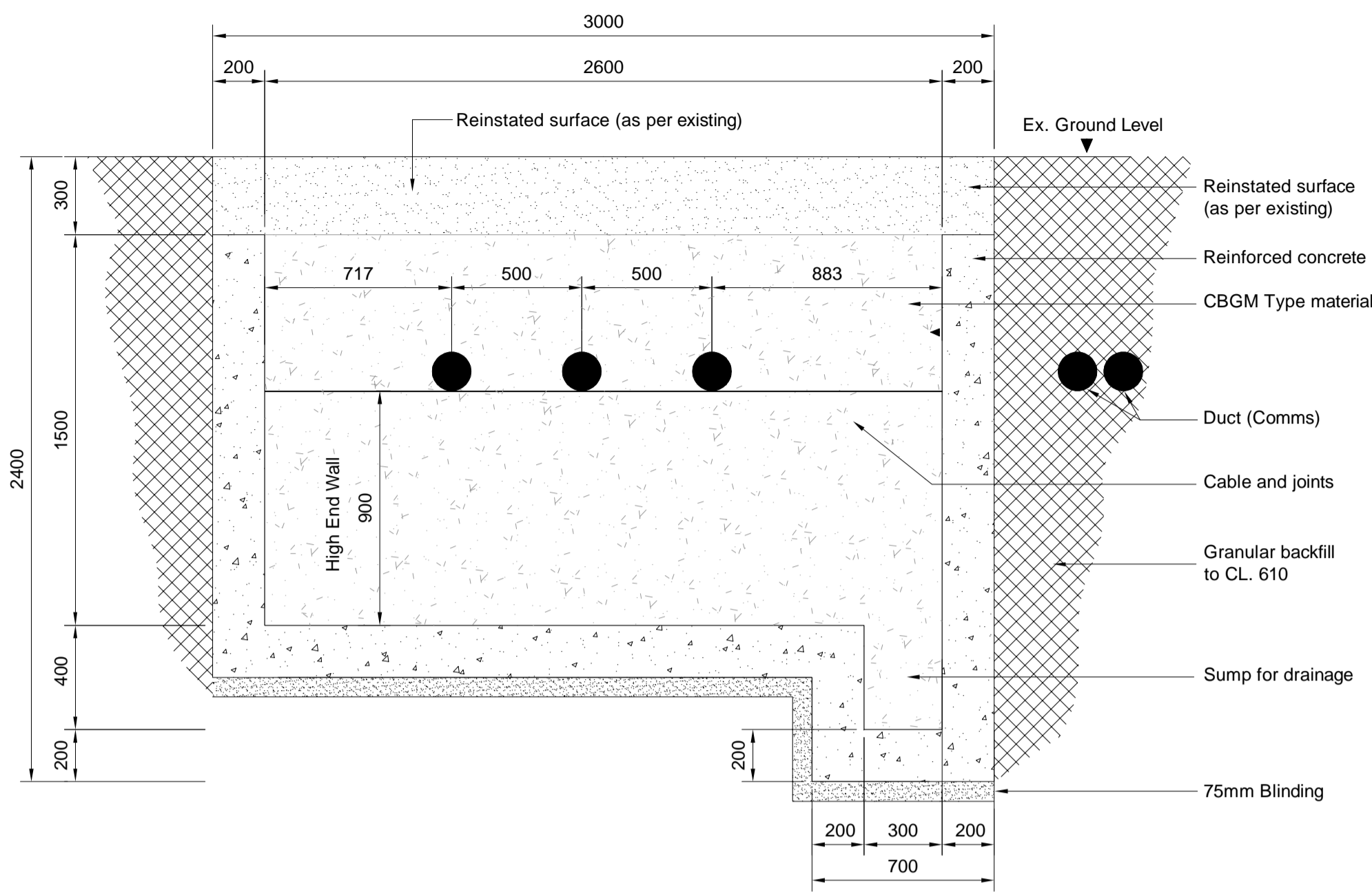
Section A-A 1:20
